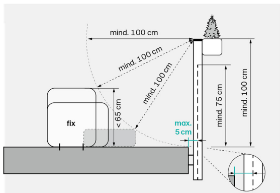
Abbildung 13 Geländer - Pflanztröge und Möbel
