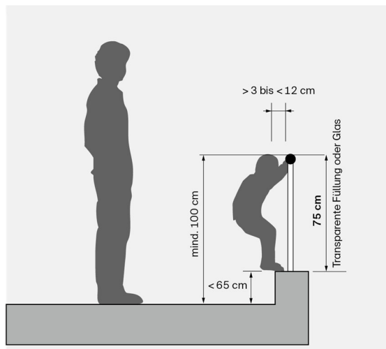
Abbildung 5 Geländer mit Füllung
